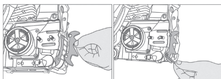
Установка упора
